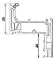
Dormant rénovation aile de 40 mm
