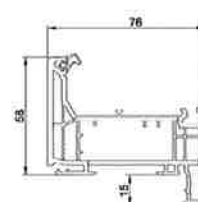
Dormant applique aile de 15 mm
