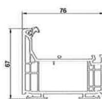
Dormant tunnel, embrasure, feuillure
