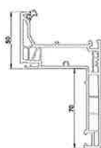
Dormant rénovation aile de 70 mm
